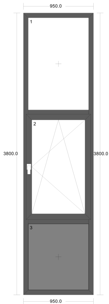
8. једнокрилни прозор са фиксним деловима 950x3800
