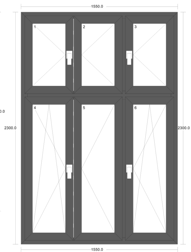
4. шестокрини прозор 1550x2300
