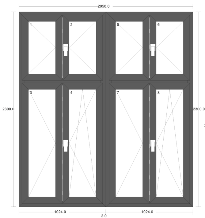
3. осмокрилни прозор 2050x2300
