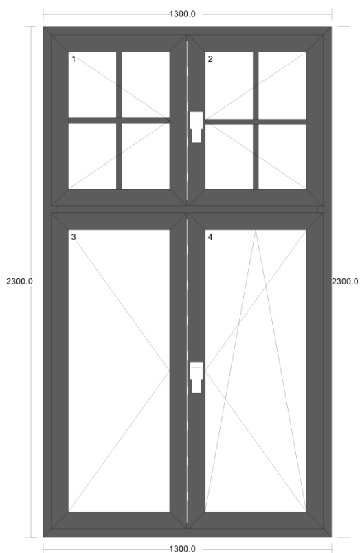
1. четворокрилни прозор 1300x2300
