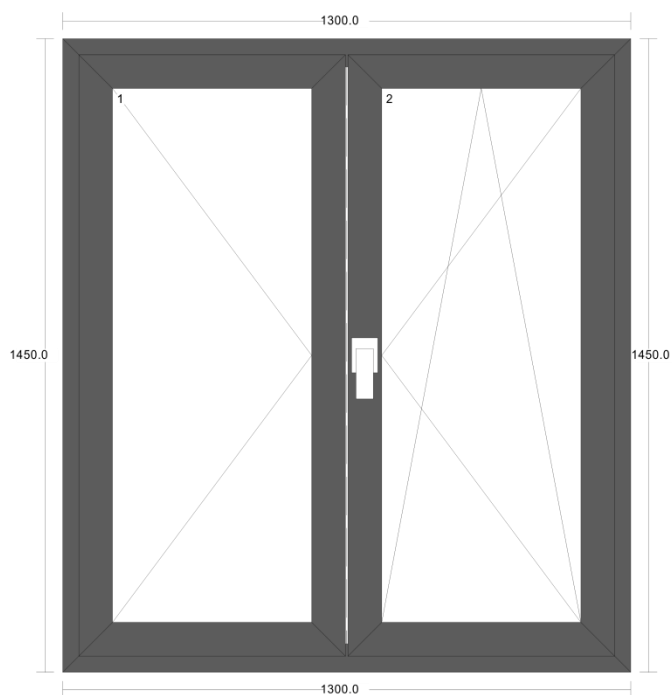
2. двокрилни прозор 1300x1450
