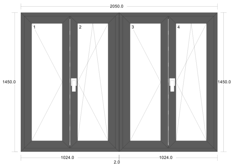
5. четворокрилни прозор 2050x1450
